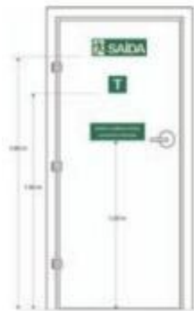
Sinalização de porta corta-fogo antipânico
